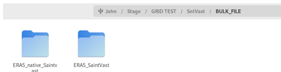
FIGURE 41 – Aperçu des dossiers générés après le téléchargement des données ERA5.
